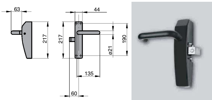
Medidas estándar de las barras. Opcionalmente pueden suministrarse para una anchura máxima de 1600 mm.
