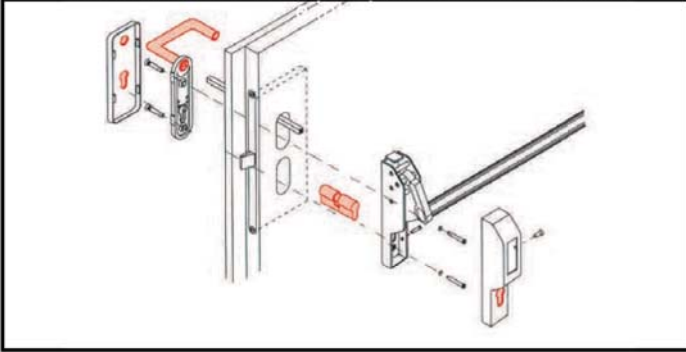
Con manilla bloqueable con llave exterior/interior
