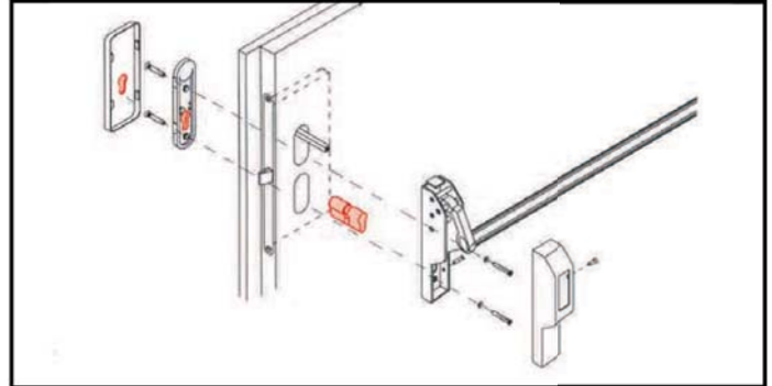
Con llave exterior
