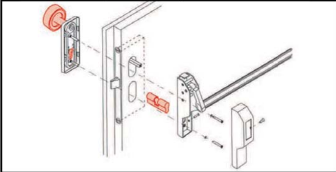
Con pomo tirador y llave exterior
