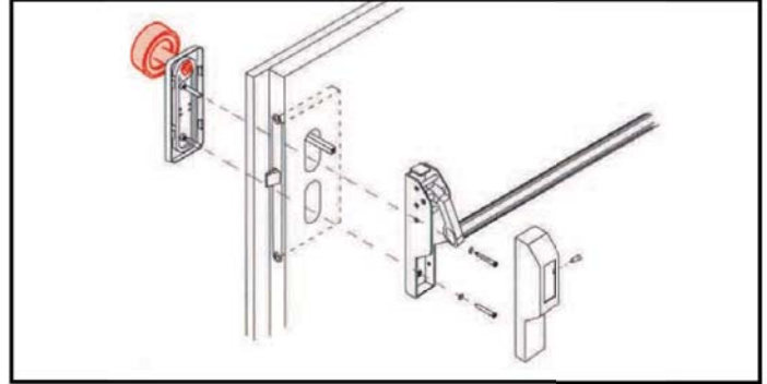
Con pomo tirador exterior
