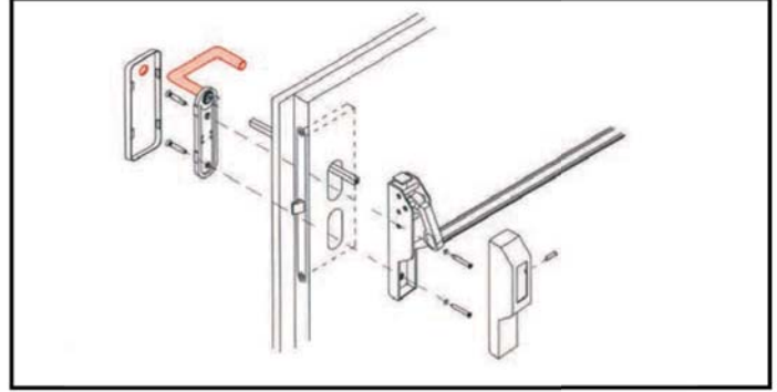
Con manilla exterior
