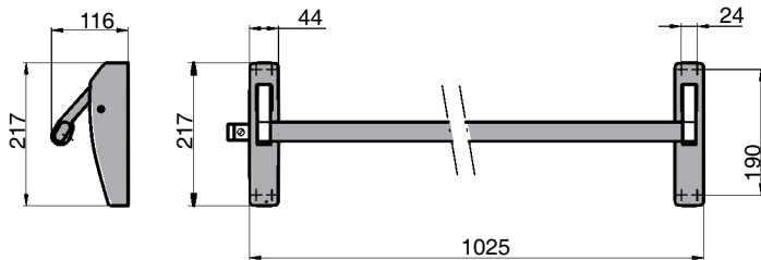
Medidas estándar de las barras. Opcionalmente pueden suministrarse para una anchura máxima de 1600 mm.
