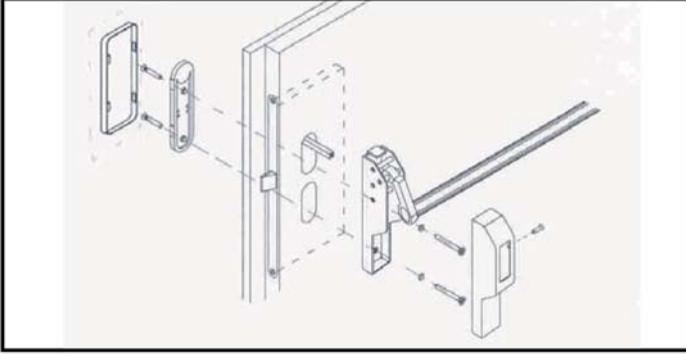
Sin accionamiento exterior
