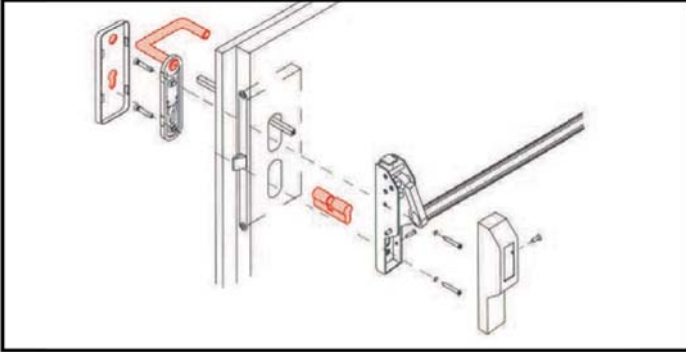
Con manilla bloqueable con llave exterior
