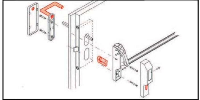
Con manilla exterior y llave interior
