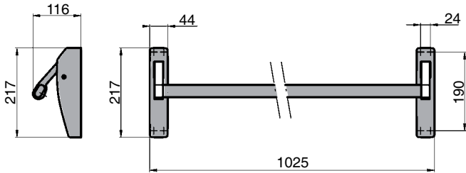
Medidas estándar de las barras. Opcionalmente pueden suministrarse para una anchura máxima de 1600 mm.
